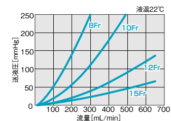
使用液体グリセリン 30%水溶液 測定時カニューレ先端は大気解放 送液特性データ(スタンダード)
