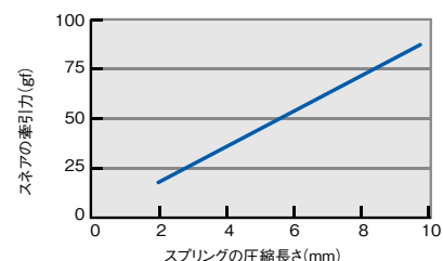
スプリングの圧縮とスネアの牽引力の関係 上記グラフは参考値で実際の牽引力を保証するものではありません。
