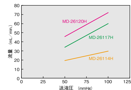
30%グリセリン水溶液の送液圧と流量の関係 上記グラフは参考値で実際の流量を保证するものではありません。
