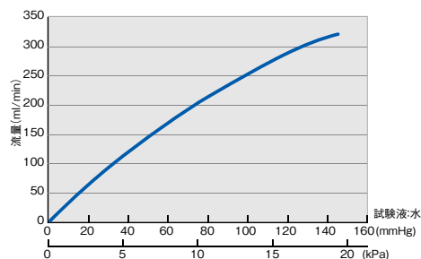
圧損と流量の関係
